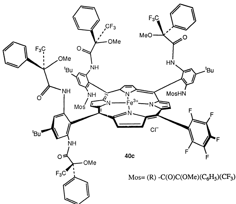
Fig. 2. Hexa-Mosher porphyrin.
